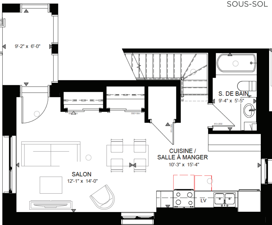
NIVEAU 1
